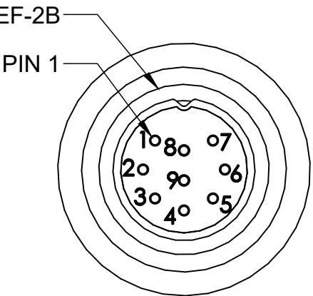
SECTION B-B SCALE 4 : 1
